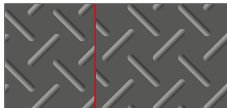
GRAFIK 6 Ansicht von oben, rote Linie = Stoß, welcher mit Fugenabdichtung gefüllt wird
