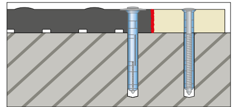
GRAFIK 7 Ansicht mit Anschlussleiste. Möglichkeit einer fugenlosen Verlegung.
