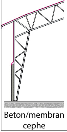
Membran cephe
