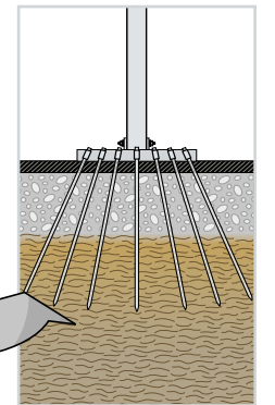
-> Yan görünüm
