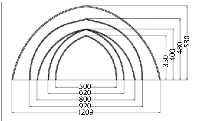
Genişlik 5 / 6,2 / 8 / 9,2 / 12m
