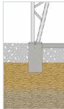
Beton şerit temel
